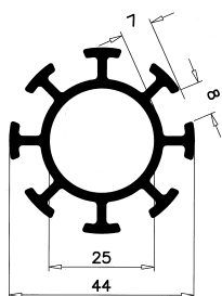
8 spors søjle monteret med stilleskrue
