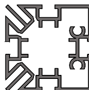
55-4-Frame-profil
