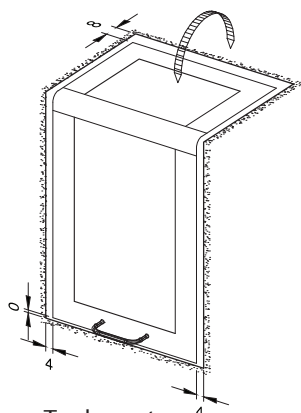
Tophængt vinkelåge
