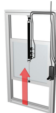
Hejselåge, pneumatisk
