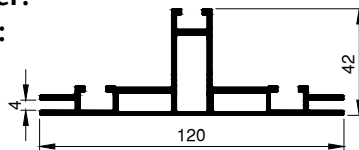
SF-44-120 ■ Til dobbeltsidet montering af grafik ■ For double sided graphics ■ Für beidseitige Grafik
