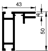
SF-44-4 ■ Til enkeltsidet montering af grafik ■ For single sided graphics ■ Für einseitige Grafik
