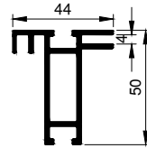
SF-44-9 ■ Mulighed for bagplade ■ Takes a back panel ■ Möglichkeit für Plattenrückwand
