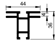
SF-36-2 ■ Til standardrammer ■ Double sided frames ■ Für Standardrahmen
