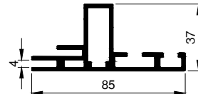
SF-44-85 ■ Til enkeltsidet montering af grafik samt bagplade ■ For single sided graphics with back panel ■ Für einseitige Grafik und Plattenrückwand
