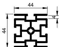
SF-44-44-4 ■ Til samling af rammer ■ For connecting frames ■ Für die Verbindung von Rahmen
