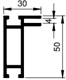
SF-44-1 ■ Til standardrammer ■ Single sided frame ■ Für Standardrahmen
