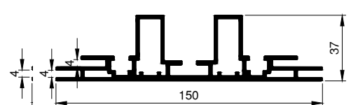
SF-44-150 ■ Til dobbeltsidet montering af grafik ■ For double sided graphics ■ Für beidseitige Grafik
