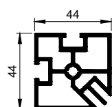
SF-44-44-2 ■ Til søjleinddækninger og kuber ■ Cubes and cladding columns ■ Für Stützenabdeckungen und Würfelbau
