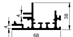
SF-44-68 ■ Til lyskasser på skinesystem ■ For light boxes on rail systems ■ Für Leuchtkästen Montiert auf Schienensysteme
