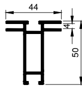
SF-44-2 ■ Til standardrammer ■ Double sided frames ■ Für Standardrahmen
