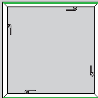
EL-FRAME-2P-F 2 x EL-PROFIL-A 2 x EL-PROFIL-B
