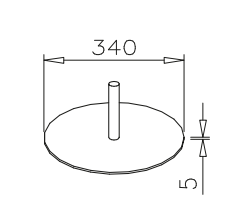
WSF-44 Fodplade med dorn. Ø340mm
