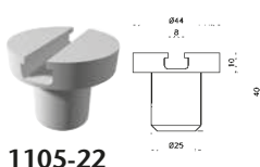
1105-22 Samleled til montering af buer på søjler. Enkelt.
