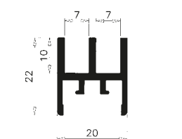
1105-13 Skydedørsprofil. Uafkor- tede længder a 5 m.
