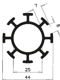
8 spors søjle monteret med stilleskrue
