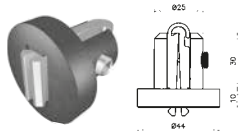
1105-21 Samleled til søjle/sarg. Sort nylon.
