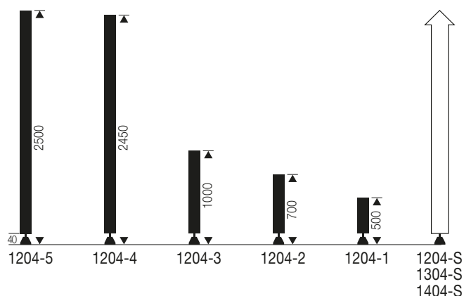
Færdige 8 spors søjler med stilleskrue Længder i mm
