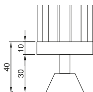
Færdige 8 spors søjler med stilleskrue Længder i mm
