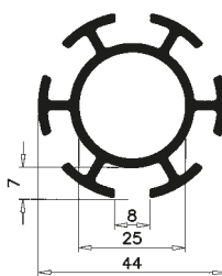
6 spors søjle monteret med stilleskrue
